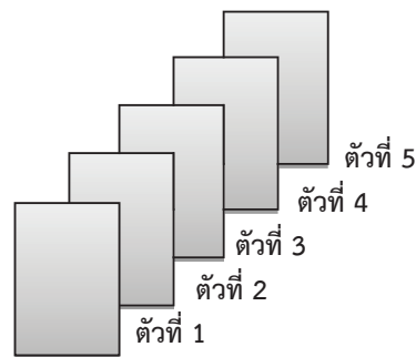
ภาพที่ 2 ทฤษฎีโดมิโน ที่มา: (Heinrich, 1978)
