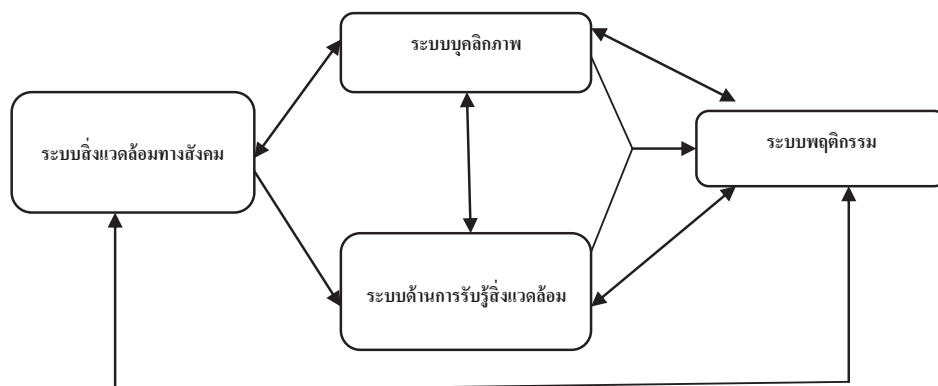
ภาพที่ 1 ทฤษฎีพฤติกรรมที่เป็นปัญหา ที่มา: (นันทา สุริรักษา, 2546, หน้า 16)
