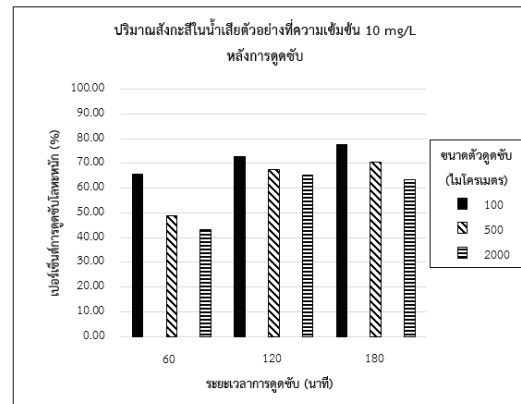
ข) \text{Zn}^{2+}
