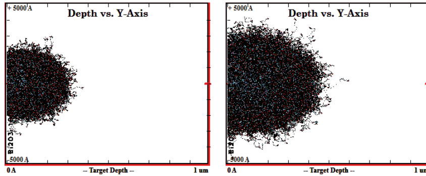
ภาพที่ 4 การจำลองอนุภาคโปรตอนผ่านเข้าไปในวัสดุแก้วที่ความหนา 1 ไมโครเมตร ที่พลังงาน 5 กิโลอิเล็กตรอนโวลต์ และ 10 กิโลอิเล็กตรอนโวลต์ ของตัวอย่างแก้วที่เติมอะตอมบิสมัทที่ความเข้มข้น 10 โมลเปอร์เซ็นต์
